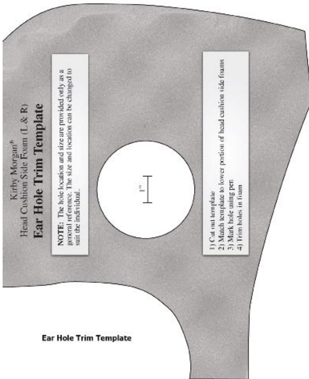
Kirby Morgan® 头垫侧面泡沫（左侧和右侧）耳机孔剪裁样板
